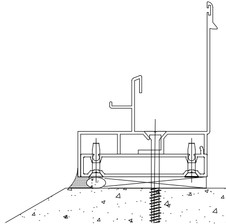
Fig 2. Instalacion con flush adapter (box)
