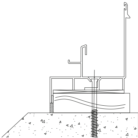
Fig 1. Instalacion sobre wood buck
